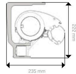
Montage contre les chevrons de toiture consoles de chevron de toiture*
