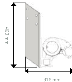
Montage contre les chevrons de toiture consoles de chevron de toiture*
